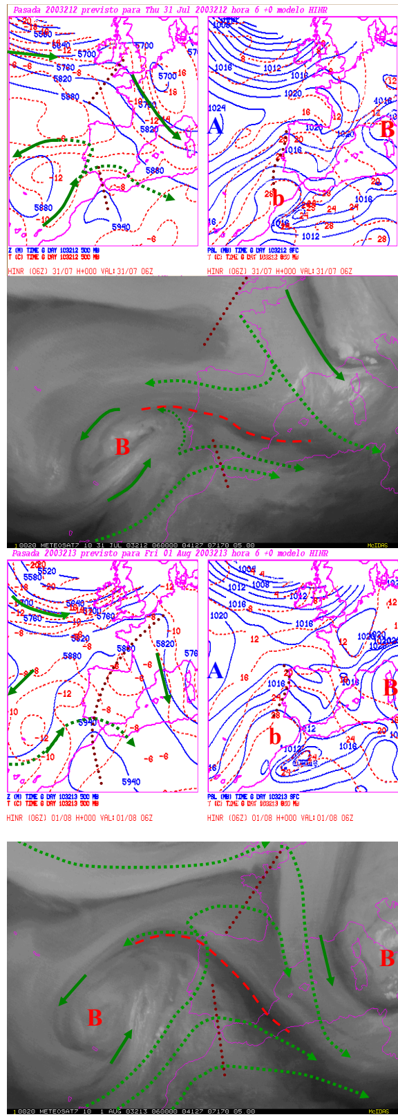
Figura 17. Análisis de 500 hPa y niveles bajos del HIRLAM-INM e imagen del canal WV062 del satélite Meteosat a las 06 UTC del 31 de julio (arriba del todo) y 1 de agosto de 2003, geopotenciales e isobaras en líneas continuas azules, isotermas, de 850 hPa en niveles bajos, a trazos rojos. Las flechas indican los chorros (líneas continuas) y el flujo en altura (a trazos), las líneas marrones a puntos, dorsales y vaguadas invertidas, las líneas a trazos indican zonas de deformación.
