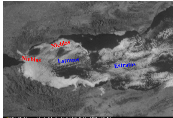
Figura 25. Imagen HRV del Meteosat de las 7:15 UTC del día 31 de julio de 2007.
